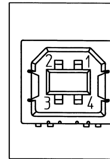
Contact No. layout (S=3/1) コンタクト番号配置図 (Plug insert face) (プラグ挿入側)
